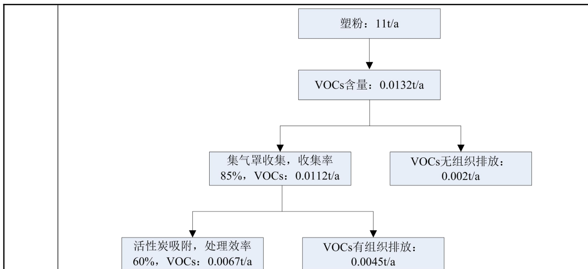
图 2-1 固化有机废气 VOCs 平衡图
