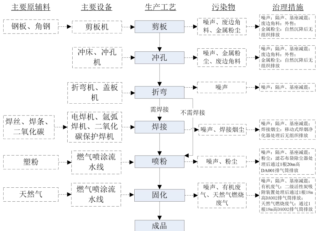
图 2-4 电缆桥架、支吊架生产工艺流程及产污位置示意图
