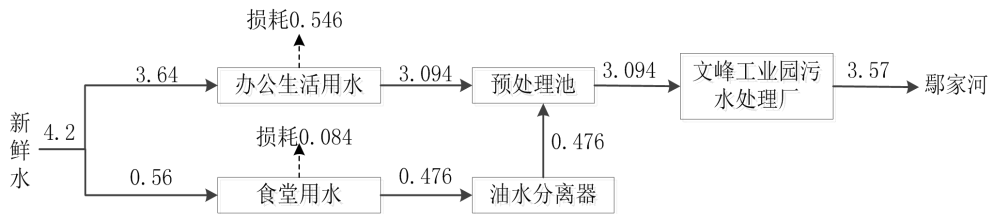
图 2-2 水平衡图 (m 3 /d)
