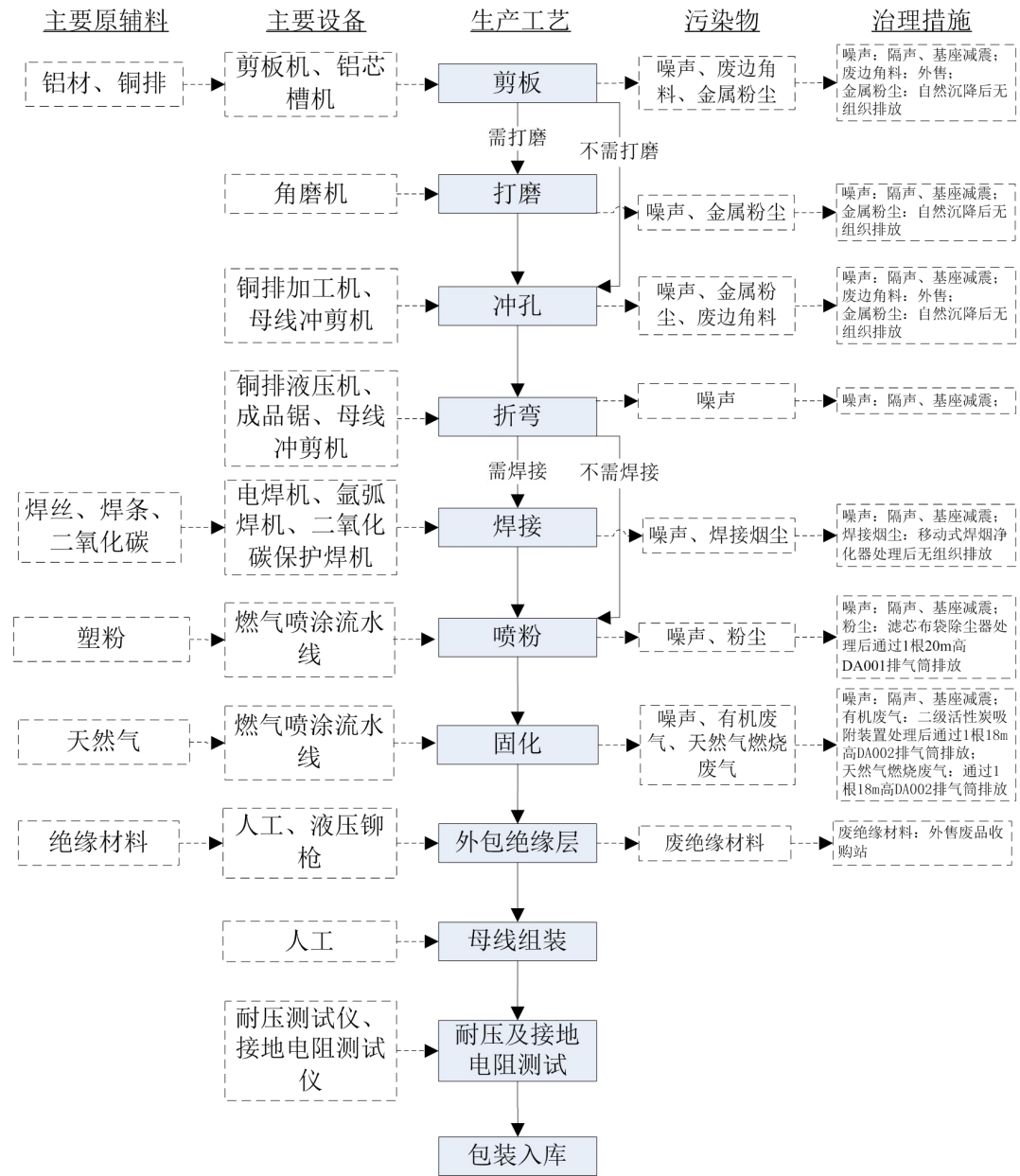
图 2-5 滤袋生产工艺流程及产污位置示意图
